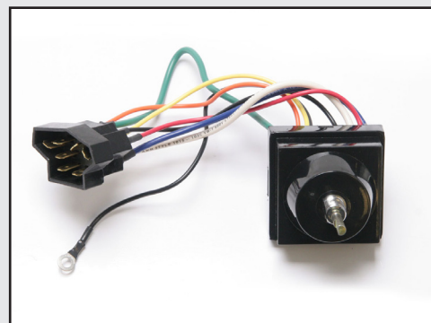
C5ZZ-17A553-V2 shown
